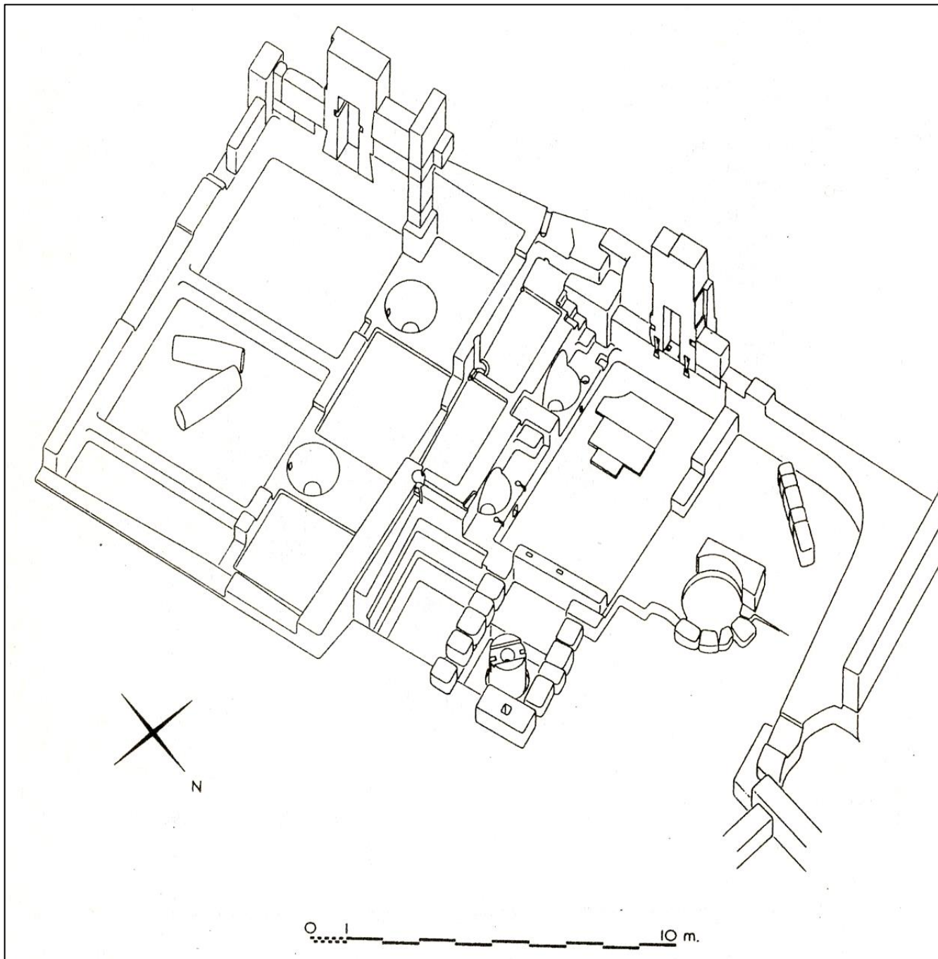
Veduta assonometrica di un impianto per la spremitura delle olive nella regione del Belus
