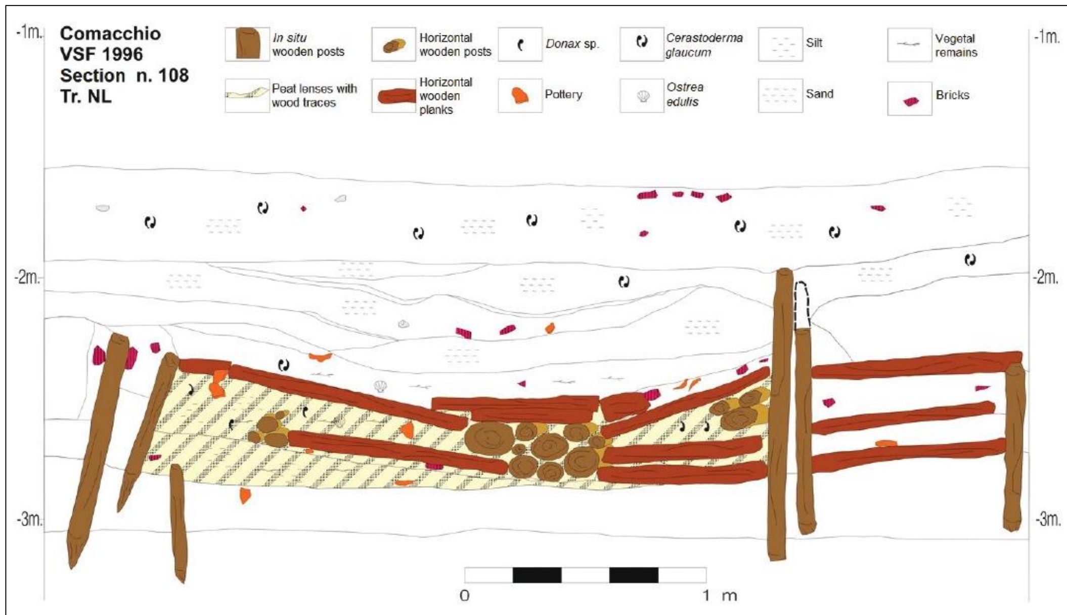
Comacchio, strutture in legno pertinenti al porto altomedievale
