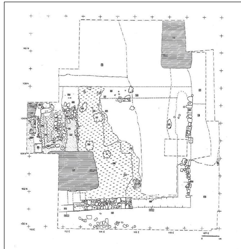
Venezia, Olivolo – San Pietro di Castello, strutture spondali ed edifici lignei
